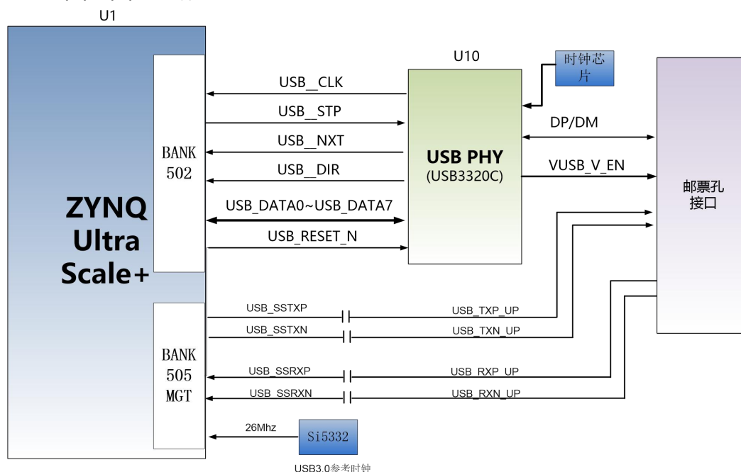
图 8-1 USB3.0 示意图
