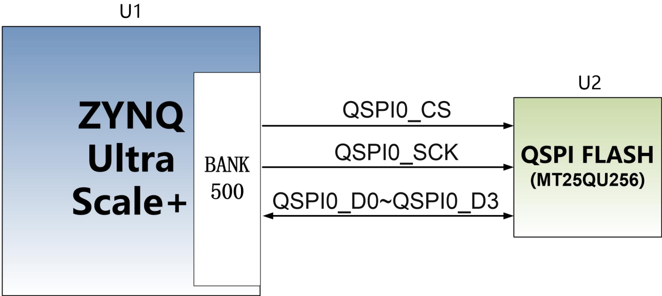
图 4-2 QSPI Flash 连接示意图
