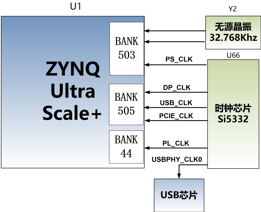
图 6-1 核心板时钟源
